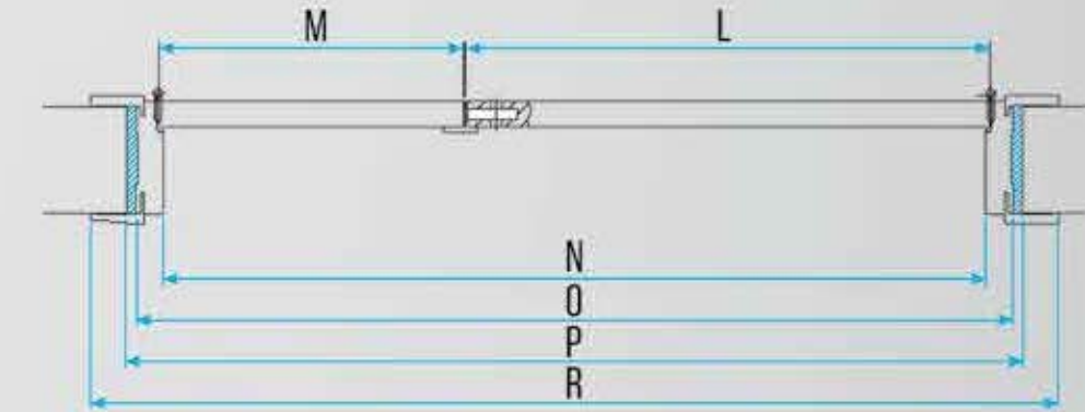
RESİM 3: SALON KAPISI GENEL KESİT
