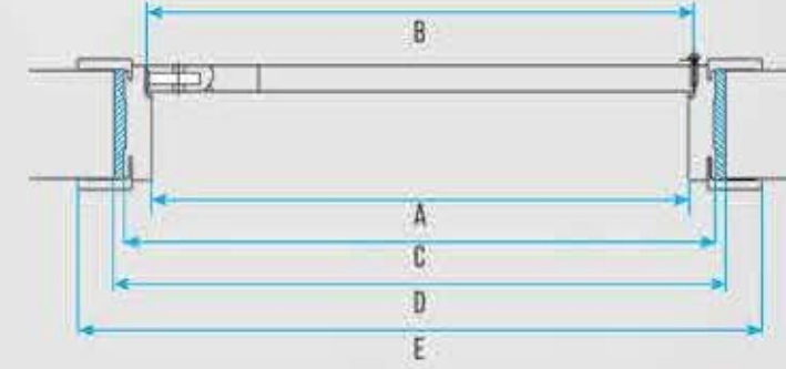
RESİM 1: KAPI GENEL KESİT
