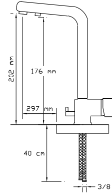
Su Arıtma Cihazı Bağlantılı Mix Eviye Batarya (Üç girişli ve çift çıkışlıdır.) 2423
