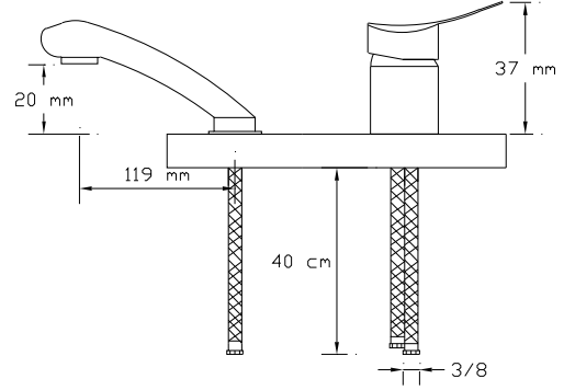
Mix Ankastra Berber Bataryası 083
