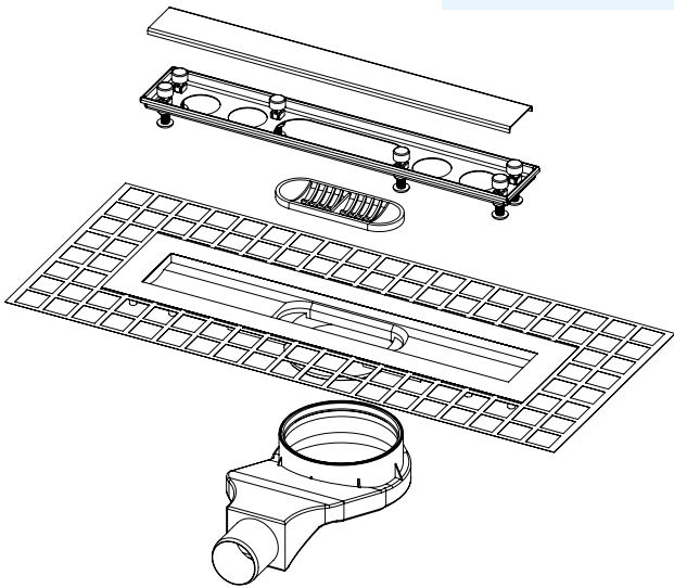
Perspektif
