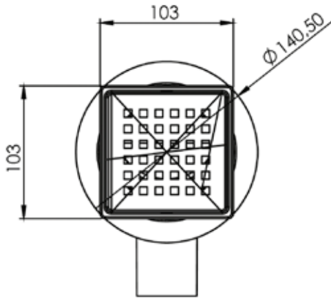
Perspektif
