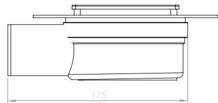
Yan Görünüm
