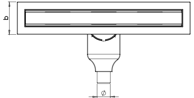
Yan Görünüm
