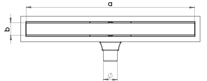
Üst Görünüm
