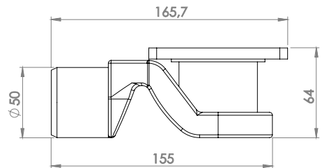
Yan Görünüm
