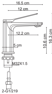
FS-8106 Osmanlı Bataryası Faucet
