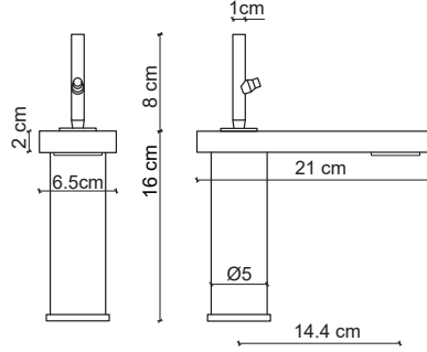
FA-8025 Yüksek Lavabo Bataryası Tall Faucet
