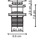
DR-10A Altın Sifon Üst Takımı Gold Pop-Up
