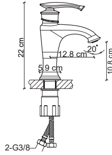
FM-1115 Lavabo Bataryası Faucet
