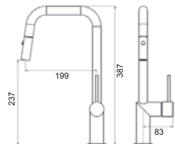
VM-2145 Vario Pull Out Kitchen Mixer - Matt Black Eviye Bataryası - Mat Siyah
