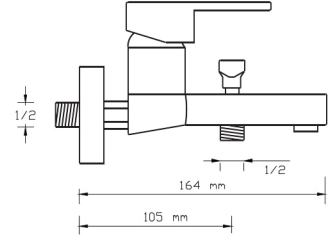
Mix Banyo Bataryası (Altın PVD İnci Parlak Siyah)
