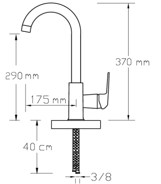
Mix Eviye Bataryası (Mat Antrasit Gri) (Döküm Gövde)
