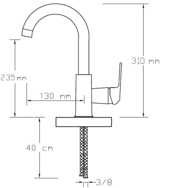
Mix Lavabo Bataryası (Mat Beyaz - Rose Altın PVD) (Döküm Gövde)
