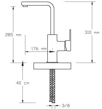
Mix Eviye Bataryası (Döküm Gövde) (Duman Gri)
