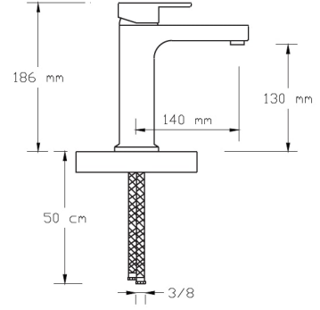
Mix Yüksek Lavabo Bataryası (Altın PVD İnci Parlak Siyah)
