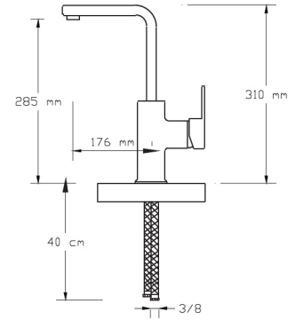
Mix Eviye Bataryası (Döküm Gövde) (İnci Derin Mavi)
