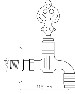
Osmanlı Musluğu (Antik Siyah) Aç-Kapa Salmastra (Perlatörlü) 2318
