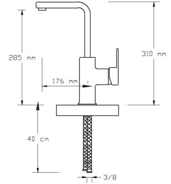
Mix Eviye Bataryası (Döküm Gövde) (Altın PVD İnci Parlak Siyah)
