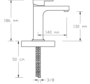
Mix Yüksek Lavabo Bataryası
