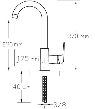
Mix Eviye Bataryası (Krom - Mat Siyah) (Döküm Gövde)
