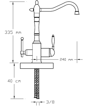
Su Arıtma Cihazı Bağlantılı Mix Eviye Bataryası (Rose Altın PVD) (Üç girişli ve çift çıkışlıdır.)
