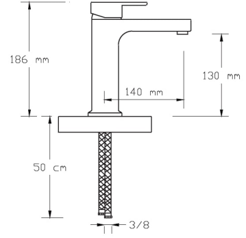
Mix Yüksek Lavabo Bataryası (İnci Parlak Siyah)
