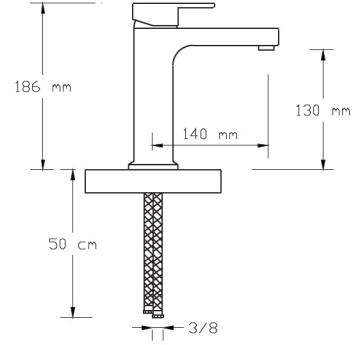
Mix Yüksek Lavabo Bataryası (Rose Altın PVD)
