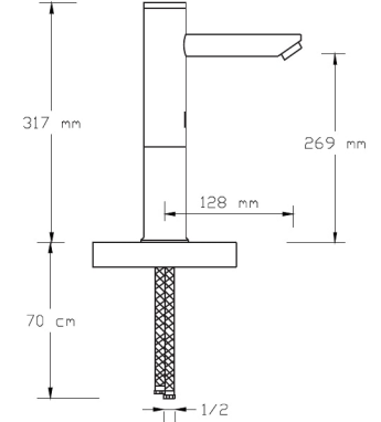
Fotoselli Çanak Lavabo Bataryası (Tek Su Girişli)
