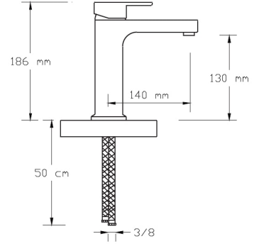
Mix Yüksek Lavabo Bataryası (İnci Derin Mavi)
