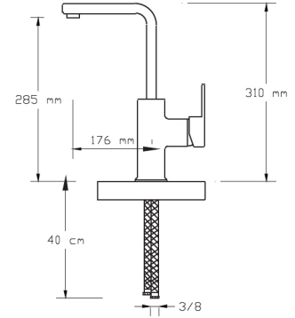
Mix Eviye Bataryası (Döküm Gövde) (Mat Siyah- Altın PVD)
