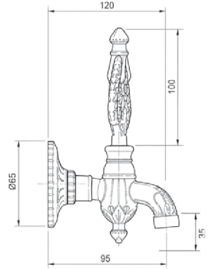
Osmanlı Musluğu, Aç-Kapa Salmastra Gizli Perlatörlü (Saten)
