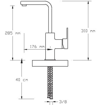
Mix Eviye Bataryası (Döküm Gövde) (Antrasit Gri)
