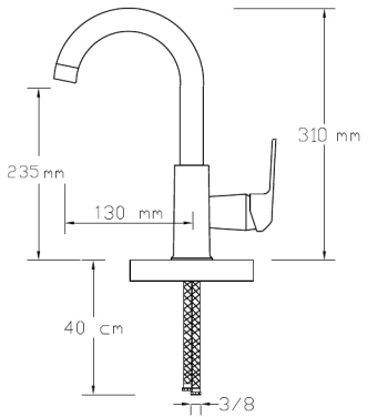
Mix Lavabo Bataryası (Krom - Mat Siyah) (Döküm Gövde)
