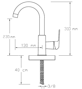
Mix Lavabo Bataryası (Krom - Rose Altın) (Döküm Gövde)
