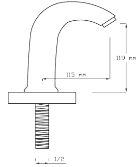
Fotoselli Lavabo Bataryası (Mat Antrasit Gri / Tek Su Girişli) 067 AG
