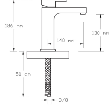
Mix Yüksek Lavabo Bataryası
