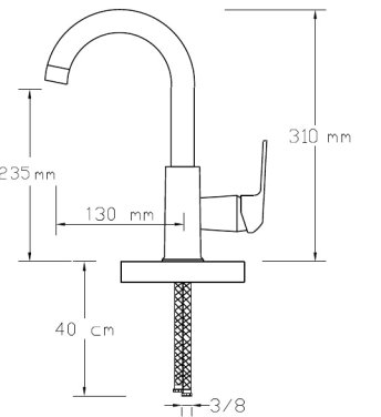
Mix Lavabo Bataryası (Mat Antrasit Gri) (Döküm Gövde)
