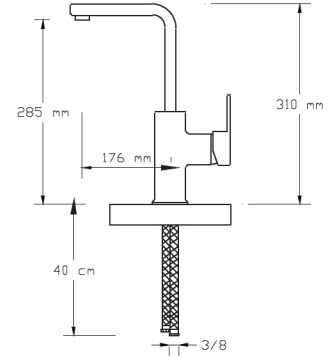
Mix Eviye Bataryası (Döküm Gövde) (Rose Altın PVD)
