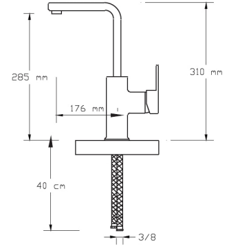
Mix Eviye Bataryası (Döküm Gövde) (Mat Siyah - Rose Altın PVD)
