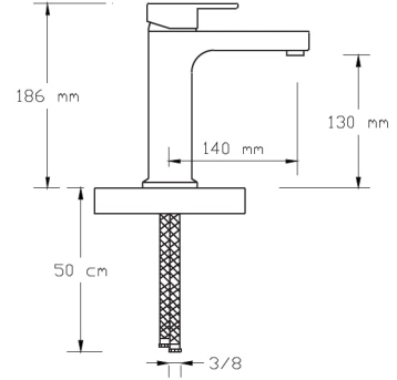
Mix Yüksek Lavabo Bataryası (Mat Siyah- Altın PVD)
