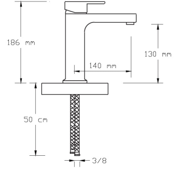
Mix Yüksek Lavabo Bataryası (Altın PVD)
