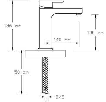
Mix Yüksek Lavabo Bataryası (Antrasit Gri)
