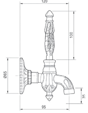
Osmanlı Musluğu, Aç-Kapa Salmastra Gizli Perlatörlü (Antik Siyah)
