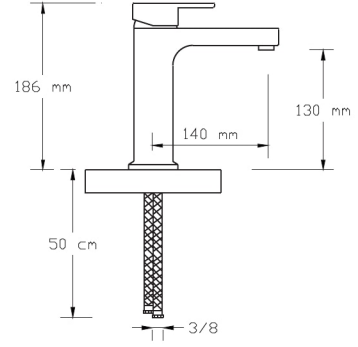
Mix Yüksek Lavabo Bataryası (Duman Gri)
