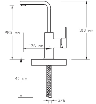
Mix Eviye Bataryası (Döküm Gövde) (İnci Parlak Siyah)
